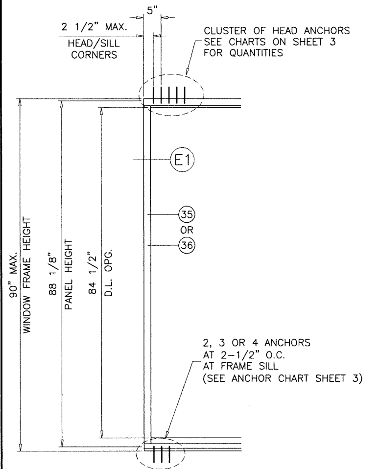
FREE STANDING JAMB OPTION W/O SIDE JAMB ANCHORS
